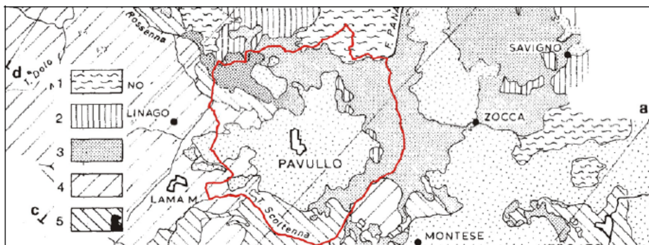
Legenda - 1) Melange di Coscogno; 2) Unità Cassio; 3) Complesso di base II; 4) Unità di Monghidoro; 5) Complesso di base I e Formazione di M. Morello. Punteggiato: depositi epiliguri; linee verticali: unità toscane e cicli messiniano-pleistocenici
